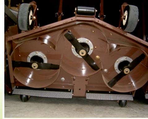
Bioclip-allemurskaus
